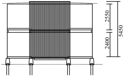
END ELEVATION
